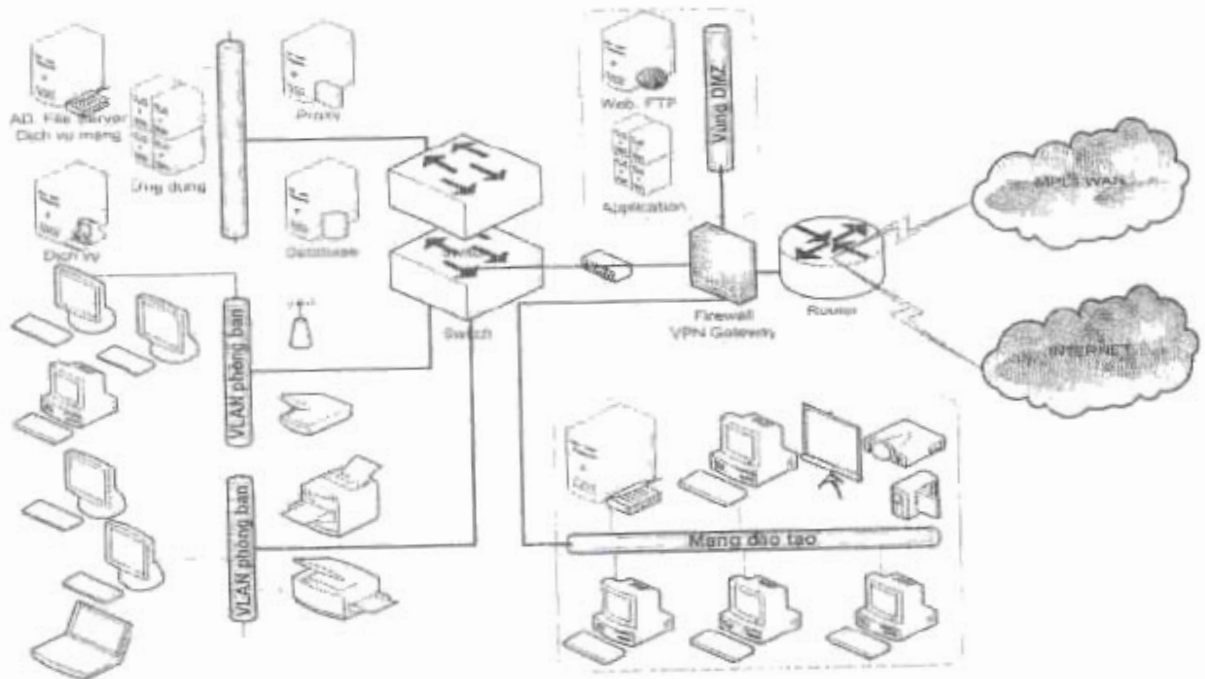
Hình 4. Sơ đồ mạng LAN tại các Trung tâm Tin học Thống kê khu vực
